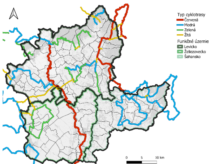
Obrázok 82 Cyklotrasy
